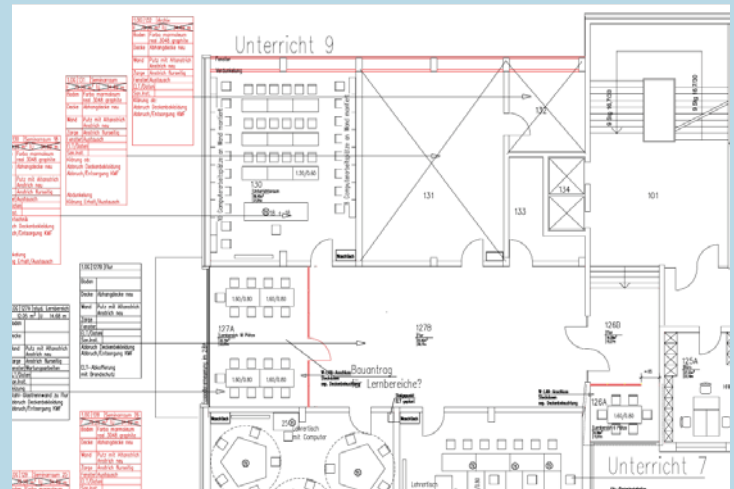
Werkplanung 1. Obergeschoss
