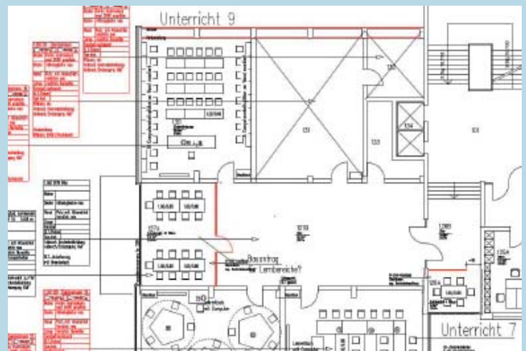
Werkplan 1. Obergeschoss
