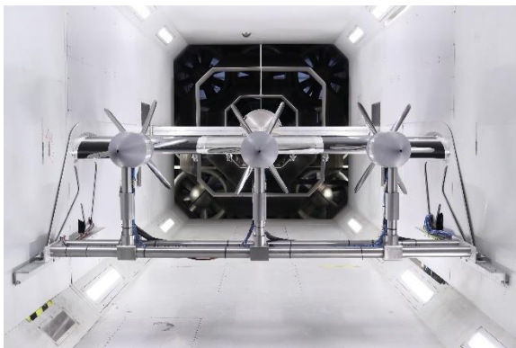
Propelleraufbau aus CICLOP im Windkanal
