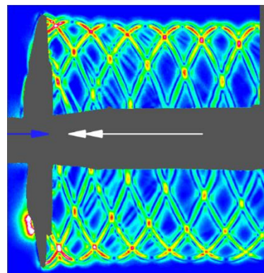
Dichtegradienten aus [1] im Propellernachlauf
