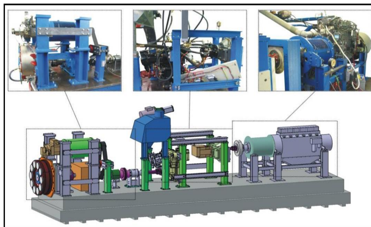
Abb. 1: Versuchsstand am IMN
